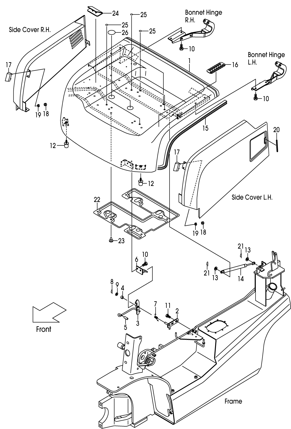
FIG.92 BONNET (F7G26420)
