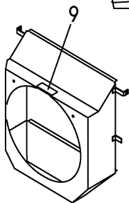
Fan Shroud
