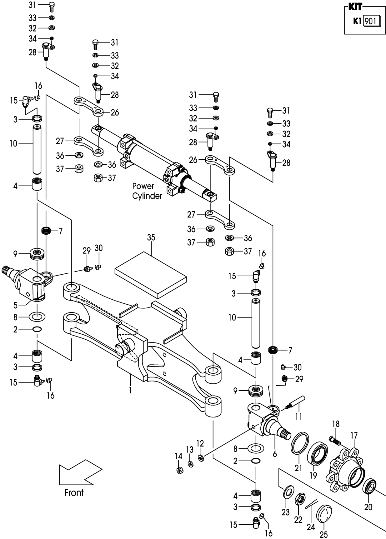
FIG.57 STEERING AXLE (F7G24310)
